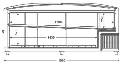
EISCF Expositor Ilha Skin Condenser Frontal
