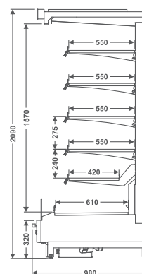
EVTVL Expositor Vertical Vision Largo
