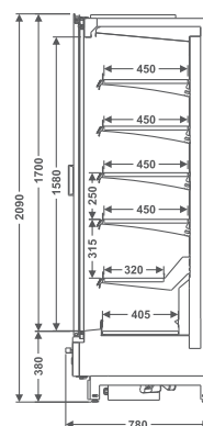
EVTVE F Expositor Vertical Vision Estreito Fechado
