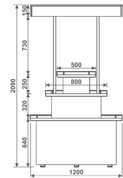
EDC NF Expositor Defumados Central Nacional Frio
