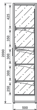
ACON NF Adega Confinados Nacional Frio
