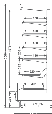
EVTVE Expositor Vertical Vision Estreito
