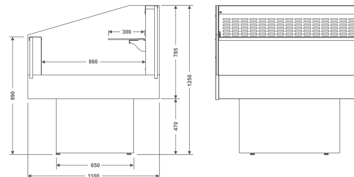
EHV1N Expositor Horizontal Vision 1 Nível
