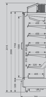
EVTVE P Expositor Vertical Vision Estreito Plug-in
