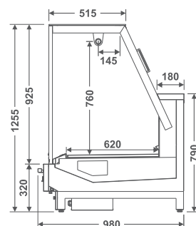
EVRVAG Expositor Vidro Reto Vision Açougue Gancheira
