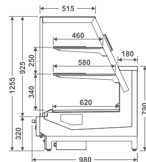
EVRVPP Expositor Vidro Reto Vision Padaria Prateleira (Refrigerado, Quente e Seco)
