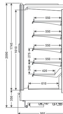
EVTVCGL Expositor Vertical Vision Congelados Largo
