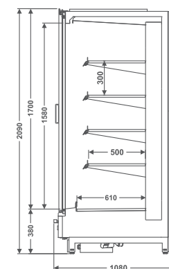
EVTVA Expositor Vertical Vision Atacado
