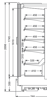
EVTVCGE Expositor Vertical Vision Congelados Estreito
