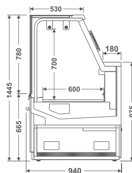
EVRVAGMA Expositor Vidro Reto Vision Açougue Gancheira Máquina Acoplada
