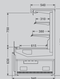
ESVUMA Expositor Semi Vertical Vision Máquina Acoplada
