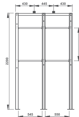
GANCHEIRA MODULAR PARA CÂMARA FRIA
