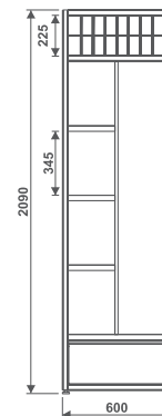
AM NF Adega Mista Nacional Frio
