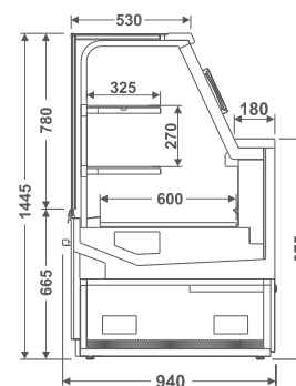
EVRVAPMA Expositor Vidro Reto Vision Açougue Prateleira Máquina Acoplada
