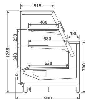
EVRVAP Expositor Vidro Reto Vision Açougue Prateleira
