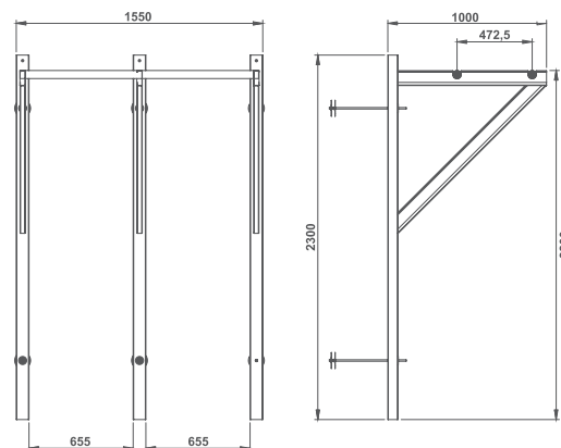
GANCHEIRA PARA DESOSSA
