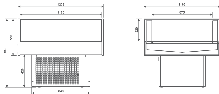
EHV Expositor Horizontal Vision
