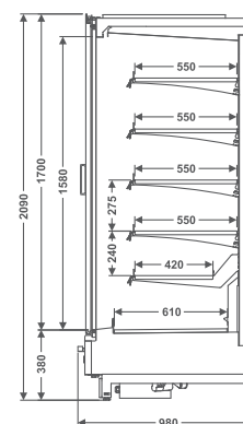
EVTVL F Expositor Vertical Vision Largo Fechado
