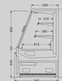
ESVAVMA F Expositor Semi Vertical Angular Vision Máquina Acoplada Fechado
