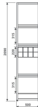
ACO NF Adega Colmeia Nacional Frio
