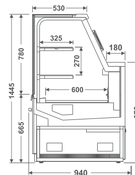
EVRVPPMA Expositor Vidro Reto Vision Padaria Prateleira Máquina Acoplada (Refrigerado, Quente e Seco)
